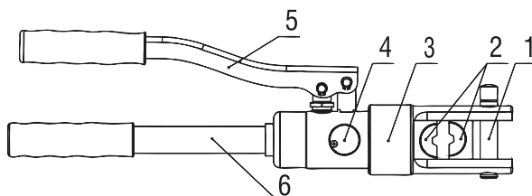
Fig.1 – Componentes
