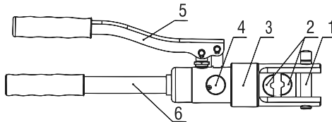
Fig.1 – Componentes
